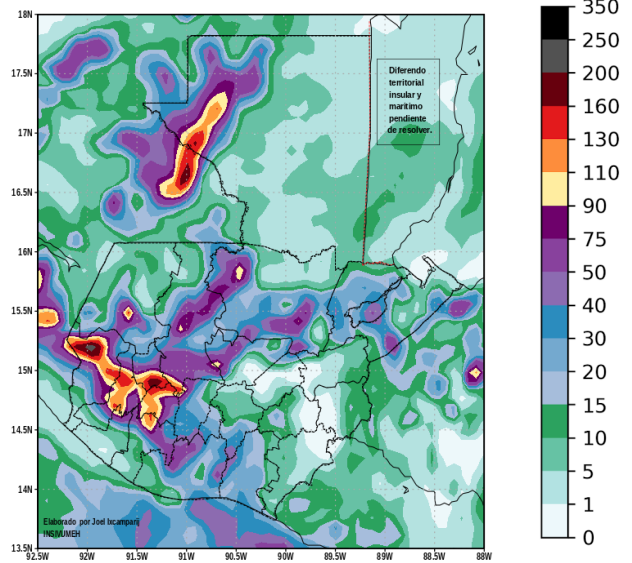
Pronostico de lluvia diaria WRF-BMJ GFS, 07JUN2024
