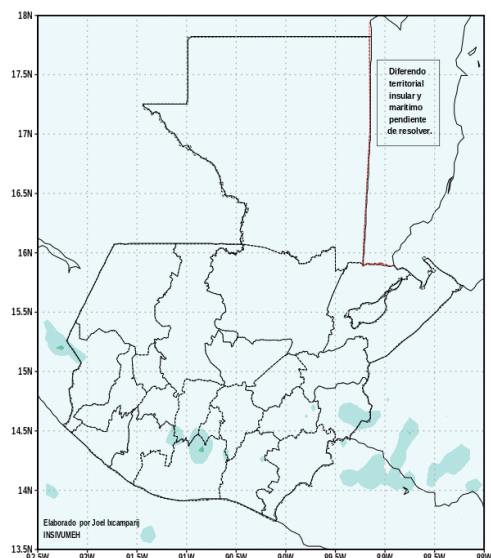
Pronostico de lluvia diaria WRF-BMJ GFS, 07MAY2024
