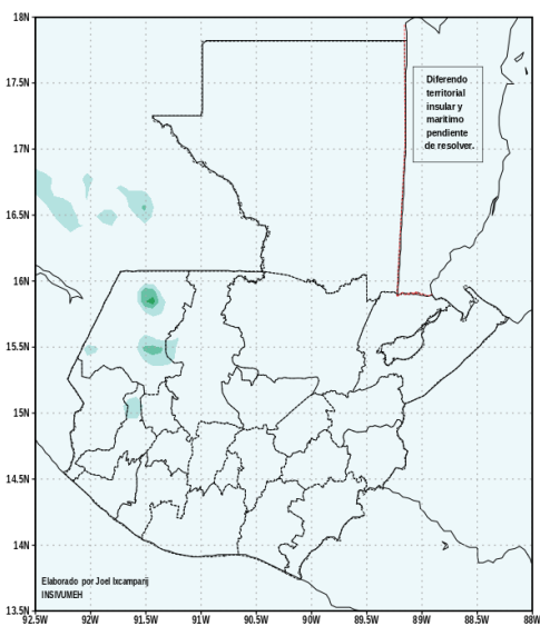
Pronostico de lluvia diaria WRF-BMJ GFS, 06MAR2024
