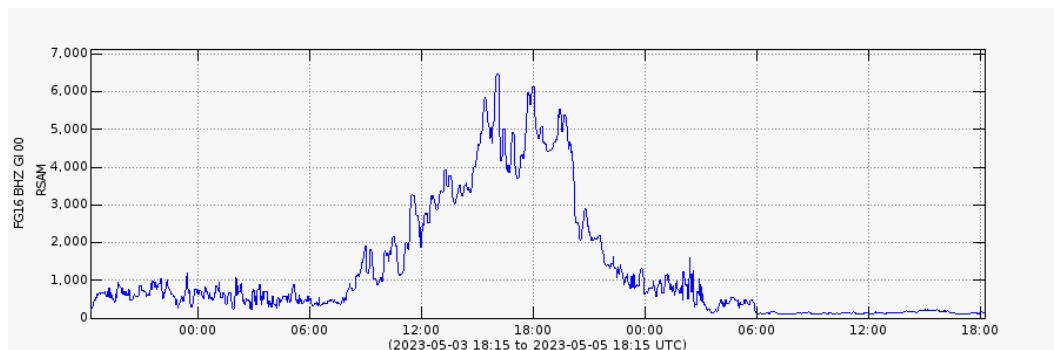
Figura 1. Gráfica de RSAM (amplitud sísmica promedio de la actividad volcánica) de las últimas 48 horas en el volcán de Fuego. Nótese la tendencia a la disminución de la actividad después de las 06:00 horas UTC (medianoche, hora local)
