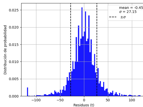
Figura 2: Histograma de los residuos temporales calculados como el horario pronosticado menos el horario observado, utilizando medias móviles de 5 horas. \sigma es la desviación estándar de los residuos y mean es el valor medio. Los datos están en minutos.
