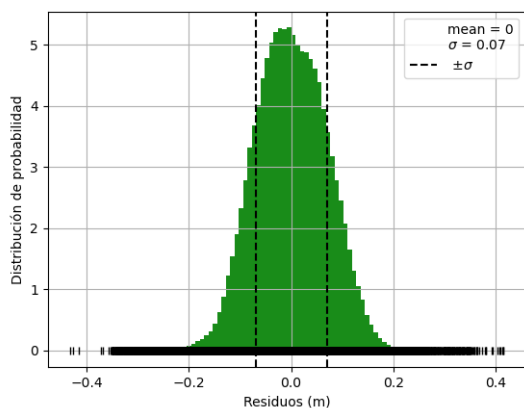
Figura 1: Histograma de los residuos calculados como el valor pronosticado menos el valor observado. \sigma es la desviación estándar de los residuos y mean es el valor medio. Los datos están en metros.
