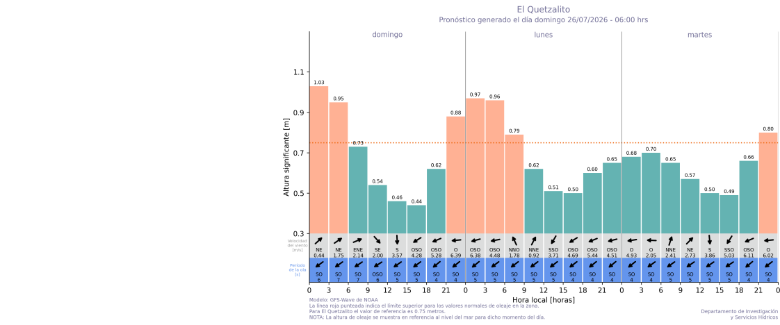
Figura 2: Pronóstico de oleaje para El Quetzalito, según el modelo GFS-Wave de NOAA.
