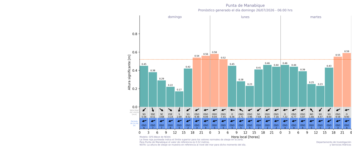
Figura 1: Pronóstico de oleaje para Punta de Manabique, según el modelo GFS-Wave de NOAA.
